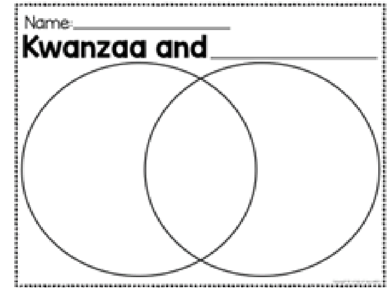
venn diagram
