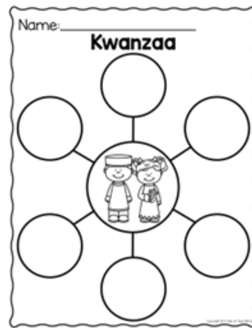
circle map
